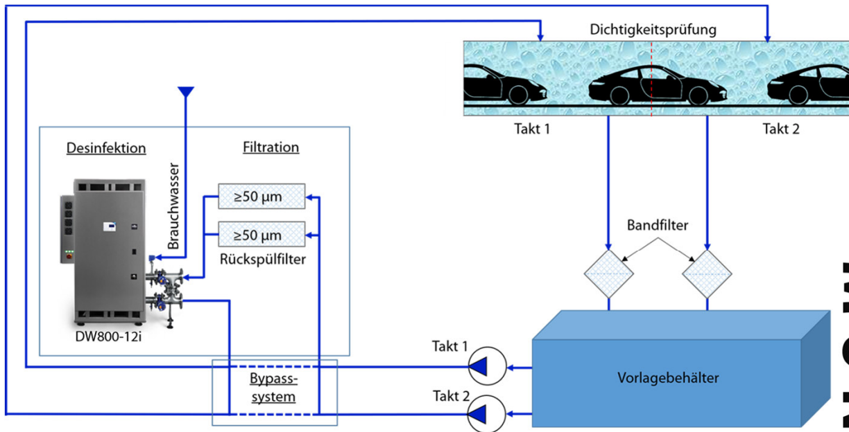
Schematische Implementierung der Wasseraufbereitung
